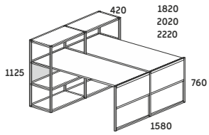
BENCH+REGAŁ 30H 2x PLECY PŁYTOWE W STANDARDZIE MONTOWANE W DOWOLNYM MIEJSCU I Z DOWOLNEJ STRONY
